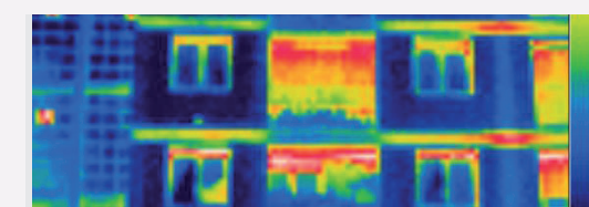
Thermographie infrarouge réalisée dans le cadre de l'accompagnement des travaux de rénovation de la résidence Marcellin Berthelot à Boulogne-Billancourt
